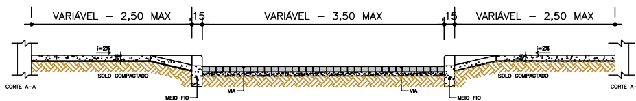
02 SEÇÃO DE TRAVESSIA ESC.: 1/75
