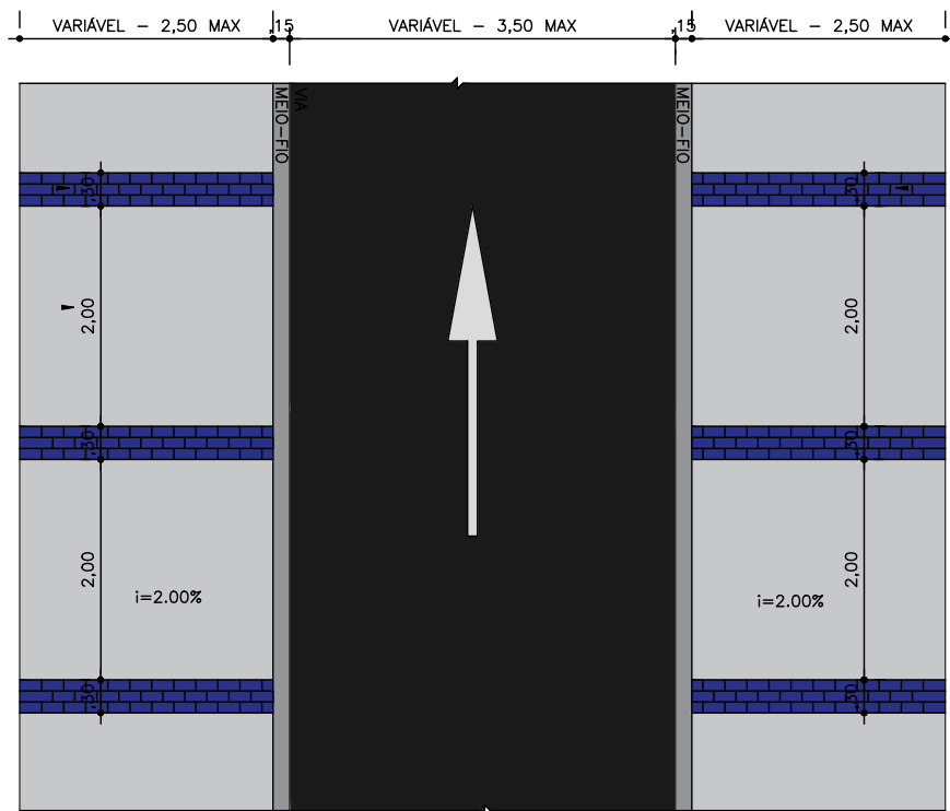
01 PLANTA BAIXA - VIA ESC.: 1/75
