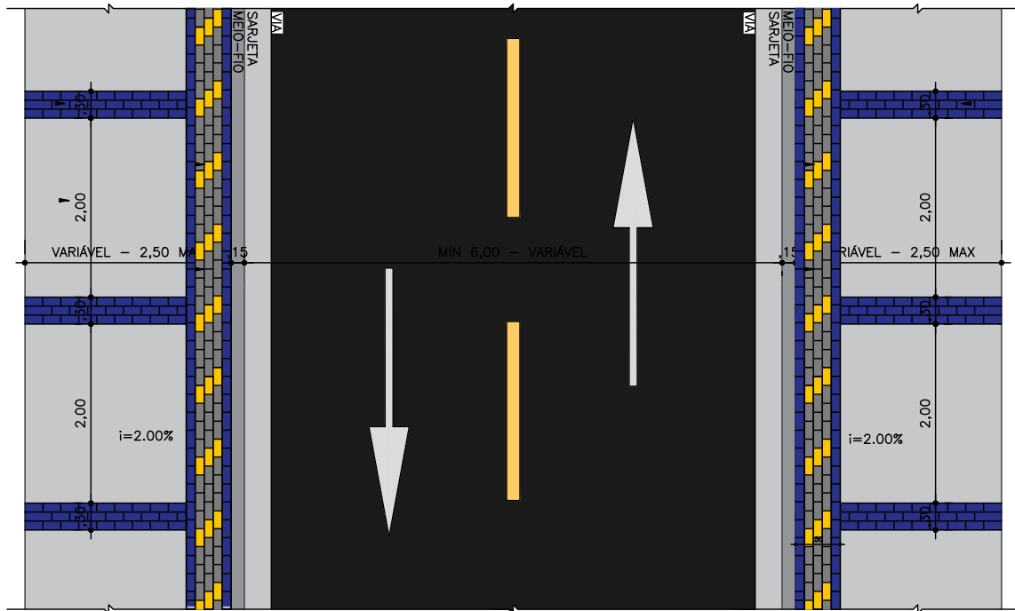
01 PLANTA BAIXA - VIA ESC.: 1/75
