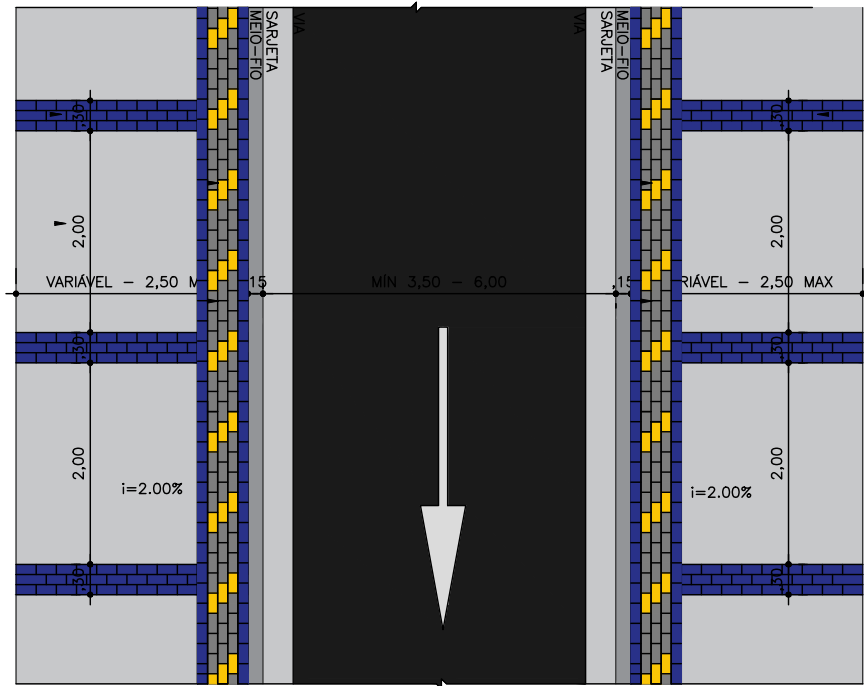
01 PLANTA BAIXA - VIA ESC.: 1/75
