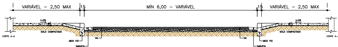
02 SEÇÃO DE TRAVESSIA ESC.: 1/75
