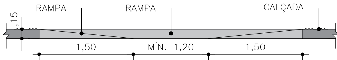
ELEVAÇÃO
