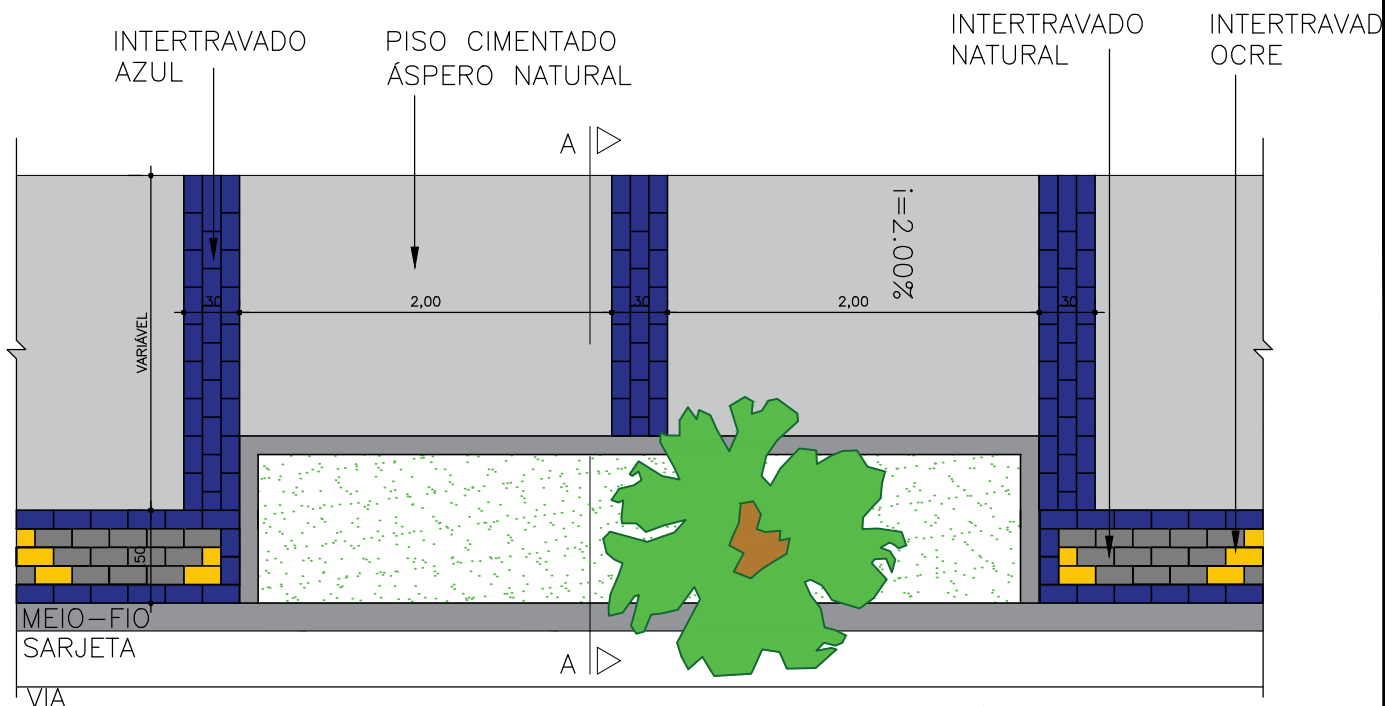
01 PLANTA BAIXA – CANTEIRO ESC.: 1/25
