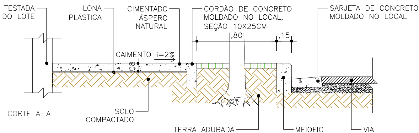
02 SEÇÃO CANTEIRO ESC.: 1/25
