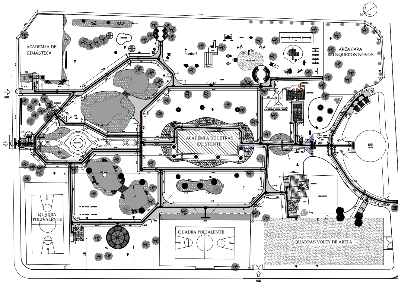
01 PLANTA DE IMPLANTAÇÃO ESC. 1:500
