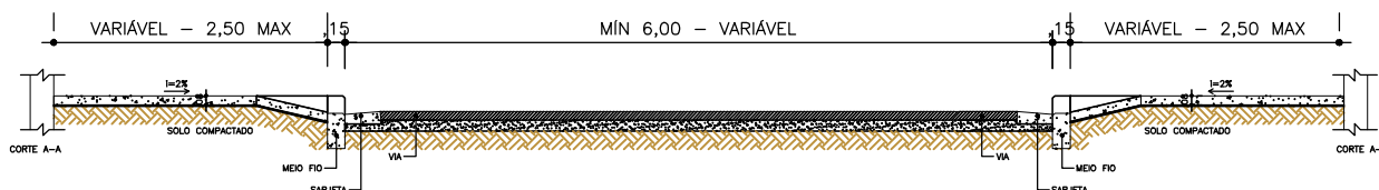
02 SEÇÃO DE TRAVESSIA ESC.: 1/75
