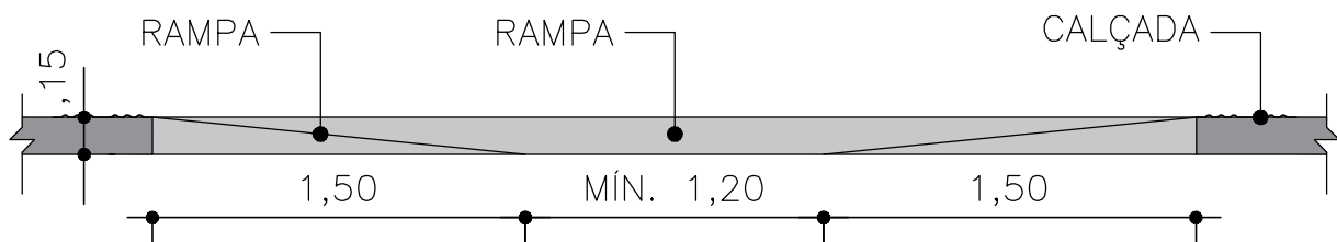
ELEVAÇÃO
